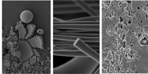
SEM slike delcev, vlaken in keramike
