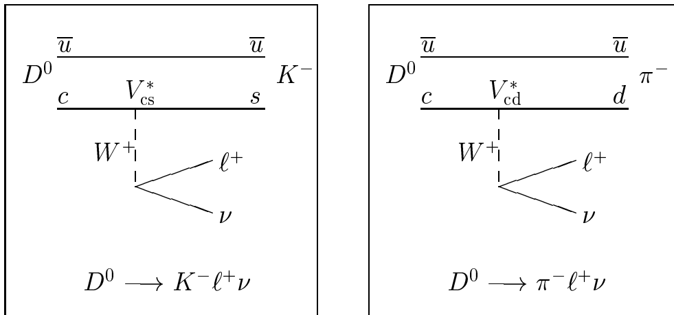
Slika 1.1: Feynmanova diagrama za semileptonska razpada mezona D^0 , katerih razmerje verjetnosti računam v tej diplomski nalogi. Pri razpadu pride do prehoda enega kvarka v drugega, zato v matričnih elementih nastopata elementa matrike CKM.
