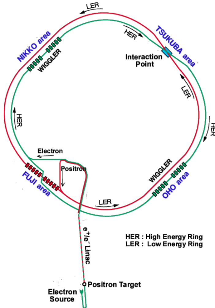
Slika 2.2: Pospeševalnik KEKB, na katerem smo zajemali podatke, uporabljene za analizo, je sestavljen iz dveh obročev s premerom približno 3 km. Po enem krožijo elektroni, po drugem pa pozitroni. Na mestu, kjer trkajo ( Interaction Point ), je nameščen detektor BELLE.
