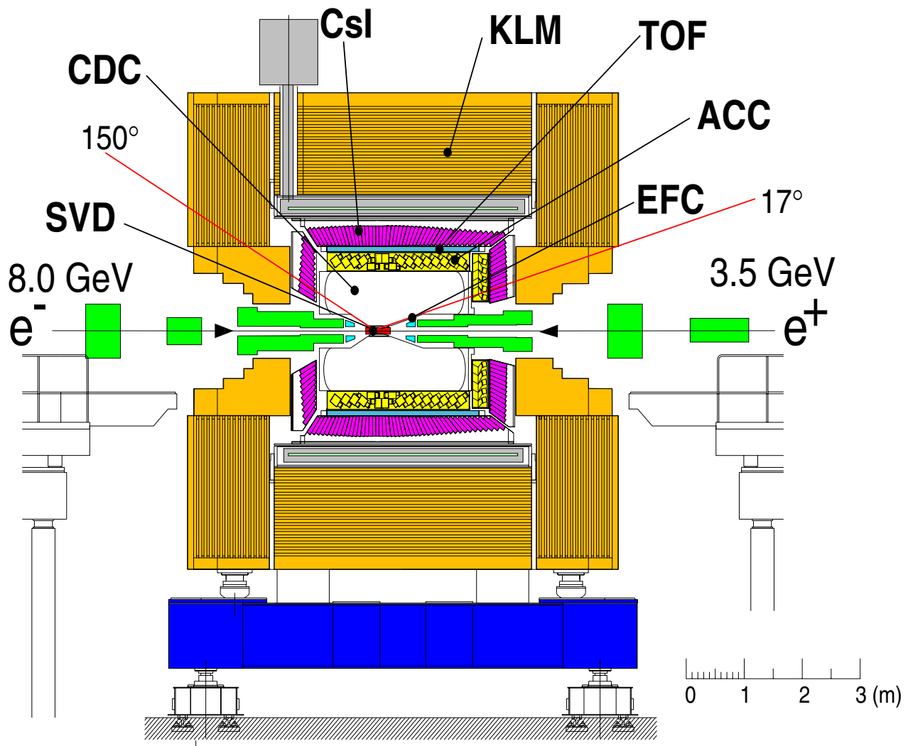
Slika 2.3: Detektor BELLE, ki detektira razpadne produkte trka e^+e^- . Sestavni deli, ki so pomembni za našo analizo, so: CDC, osrednja potovalna komora, kjer potekajo meritve gibalnih količin in identifikacija delcev, TOF, merilec časa preleta, ki služi za razločevanje med kaoni in pioni, ACC, števec Čerenkova, tudi za razločevanje med kaoni in pioni, CsI, elektromagnetni kalorimeter za identifikacijo elektronov in KLM, detektor mionov in dolgoživih mezonov K_L .
