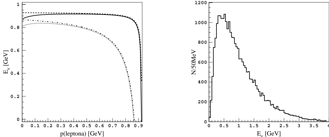
Slika 3.1: Levo: energija nevtrina v razpadu D^0 \rightarrow h^- \ell^+ \nu kot funkcija gibalne količine nabitega leptona v mirovnem sistemu D^0 v primeru, da hadron in lepton odletita v isto smer. V tem primeru lahko nevtrino odnese največ energije - tudi do 0,93 GeV. Narisane so štiri krivulje za štiri razpade, od spodaj navzgor: (pikčasto) D^0 \rightarrow K^- \mu^+ \nu_\mu , (pika-črta) D^0 \rightarrow K^- e^+ \nu_e , (polna črta) D^0 \rightarrow \pi^- \mu^+ \nu_\mu in (črtkano) D^0 \rightarrow \pi^- e^+ \nu_e . Desno: Simulirana porazdelitev nevtrinov iz razpada D^0 \rightarrow h^- \ell^+ \nu po energiji nevtrina v laboratorijskem sistemu. Ker se delec D^0 v laboratorijskem sistemu giba s hitrostjo, ki je blizu svetlobni, so energije nevtrina v tem sistemu lahko tudi znatno večje kot v sistemu delca D^0 , za katerega je narisan levi graf.
