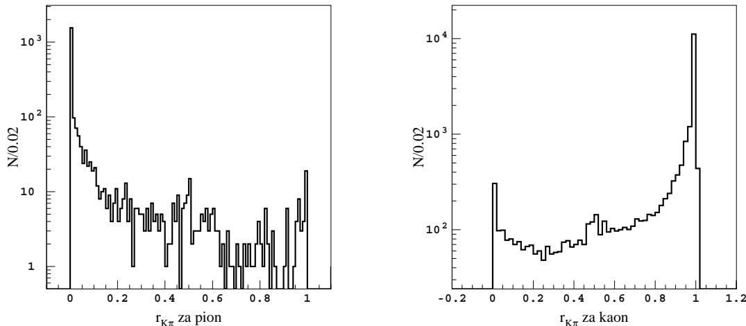
Slika 4.3: Simulirana porazdelitev po kvocientu r_{K\pi} za pione (levo) in kaone (desno). Z zahtevo r_{K\pi} < 0,2 zavrneemo 13% vseh pionov in 95% vseh kaonov iz obravnavanih semileptonskih razpadov mezona D^0 . Prepuščene delce tako sestavlja okrog 65% pionov in 35% kaonov. (To drži, če upoštevamo le pione in kaone. Lahko pa tudi elektron in še zlasti mion napačno identificiramo kot pion.) Grafa sta v logaritemski skali.
