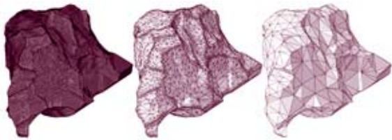
Slika 3: Primer rekonstrukcije površine kristalnega zrna (Simonovski s sodelavci). Levo je rekonstrukcija površine z največjo natančnostjo, ki jo dopuščajo meritve z difrakcijsko kontrastno tomografijo. V sredini in desno pa so različne stopnje poenostavitve površine, ki jih uporabljamo v modelih za računalniške simulacije. Poenostavitve so nujne zaradi omejenih računalniških zmogljivosti.
